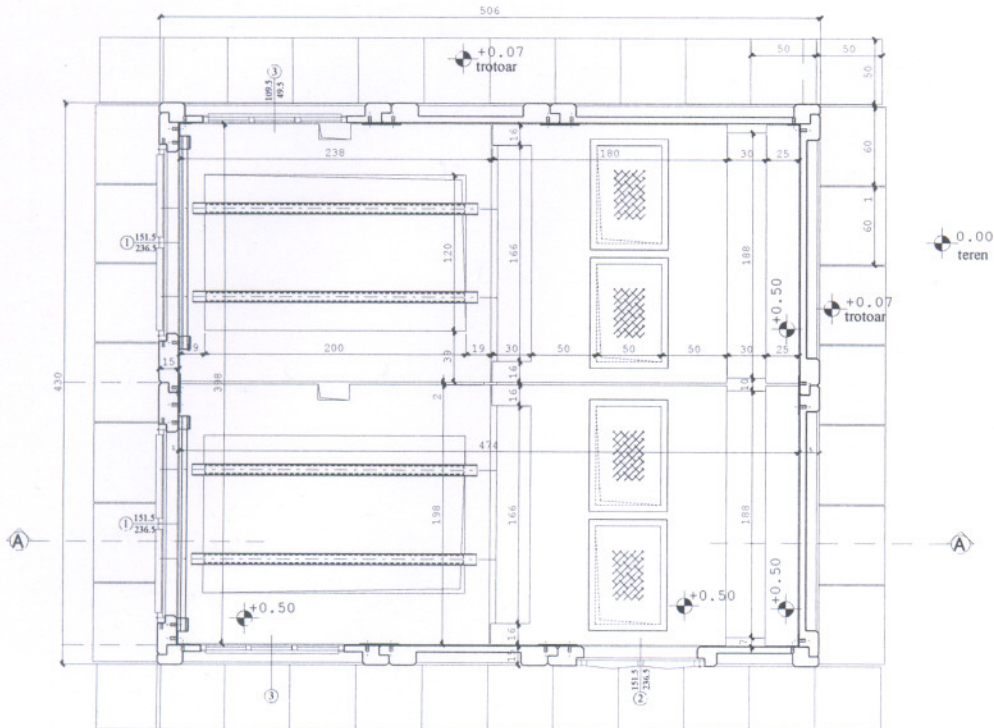
OSNOVA PRIZEMLJA
