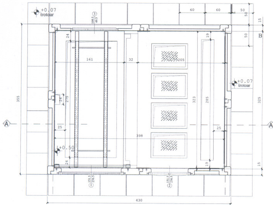
OSNOVA PRIZEMLJA
